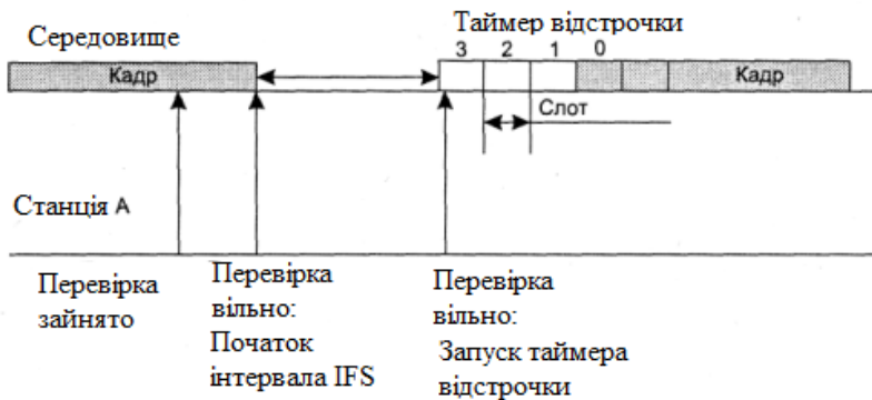
Рисунок 2.2 – Режим доступу DCF
