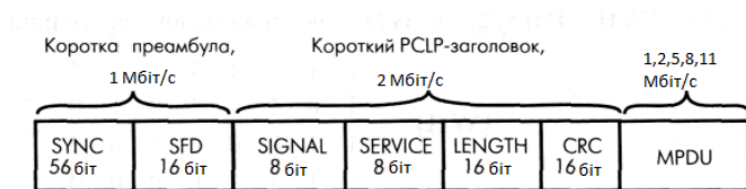
Рисунок 2.13 – Короткий заголовок кадрів мережі 802.11b
