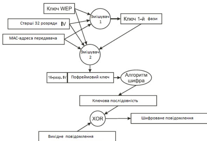
Рисунок 8.7 – Процес створення шифрованого повідомлення в WPA
