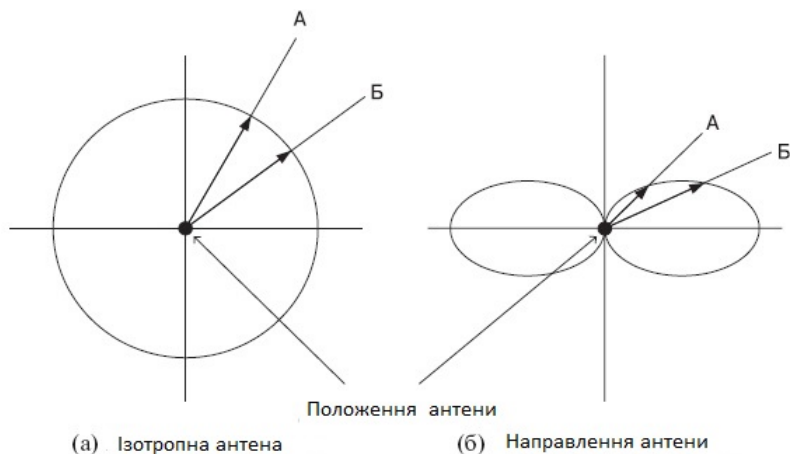
Рисунок 11.1 – Діаграми спрямованості
