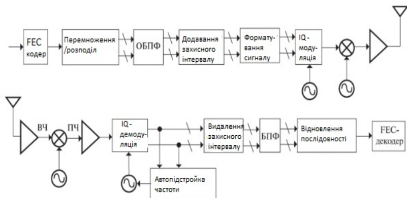
Рисунок 2.11 – Функціональна схема трактів приймання/передачі стандарту IEEE 802.11a
