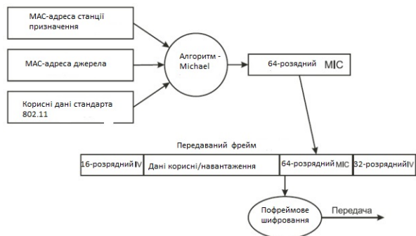
Рисунок 8.8 – Робота алгоритму Michael MIC
