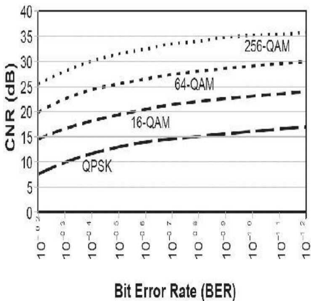
Рисунок Д.9 – Відношення CNR до BER
