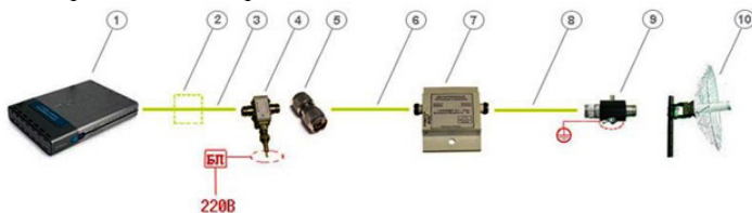
Рис. 12.6 – Антенно-фідерний тракт із підсилювачем
