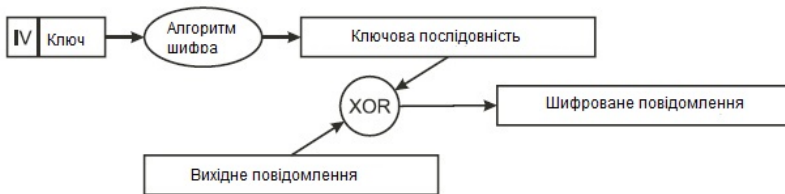
Рисунок 7.3 – Алгоритм шифрування WEP
