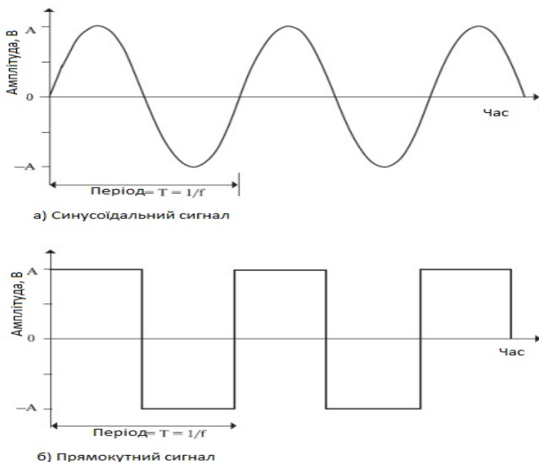
Рисунок 1.7 – Періодичні сигнали
