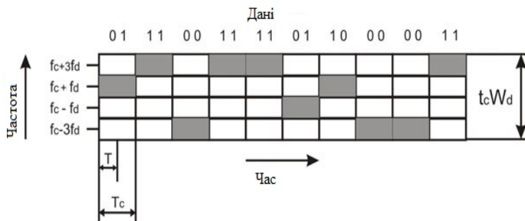
Рисунок 1.2 – Використання частоти схемою MFSK ( M = 4 )
