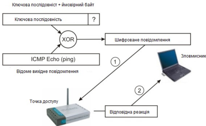
Рисунок 7.6 – «Вирощування» ключової послідовності
