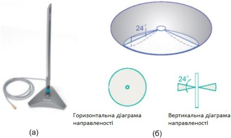
Рисунок Г.1 – Антена ANT24-0700
