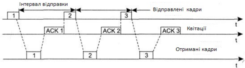
Рисунок 1.13 – Процедура запит ARQ із зупинками
