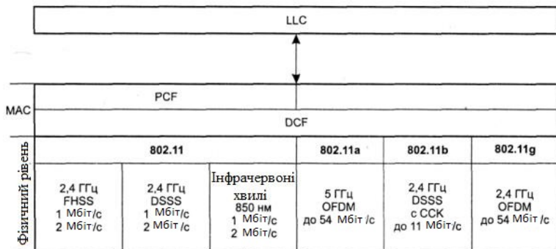
Рисунок 2.1 – Стек протоколів IEEE 802.11
