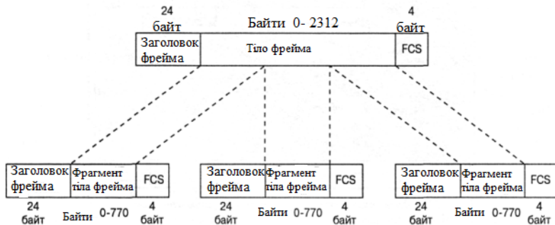
Рисунок 2.4 – Фрагментація фрейму
