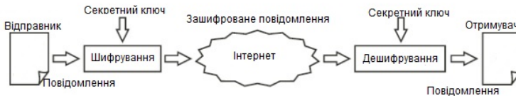
Рисунок 6.1 – Симетричне шифрування
