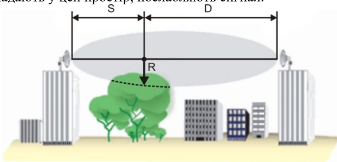
Рисунок 12.1 – Зона Френеля
