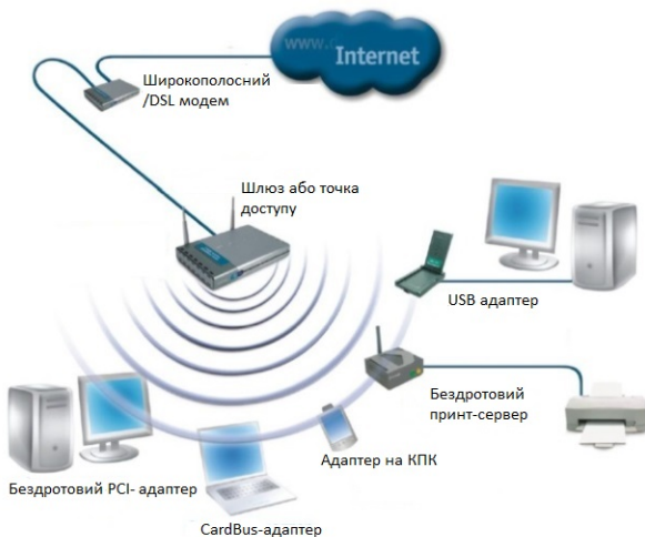
Рисунок 4.1 – Офісна мережа
