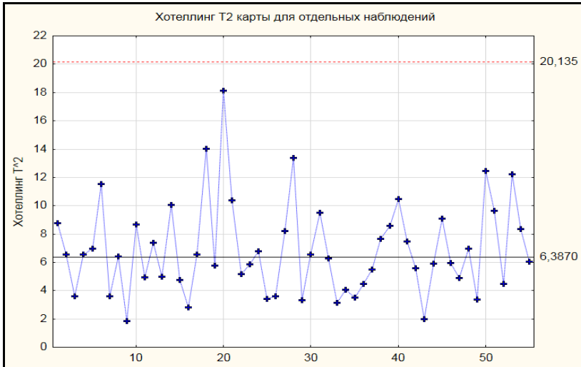
Рис. 12. Карта Хотеллінга T^2 для окремих спостережень удосконаленого процесу
