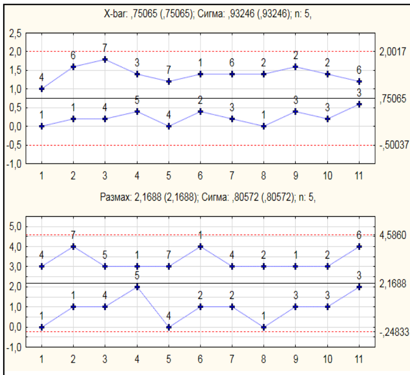
Рис. 13. Багатовимірний потік з X-bar та R-картами вдосконаленого процесу
